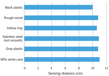
Background suppression
